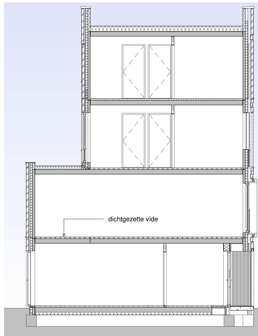
Doorsnede A-A
