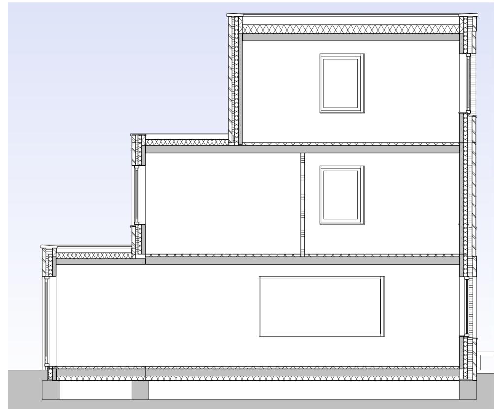
Doorsnede A-A
