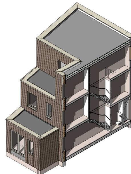
Isometrie
