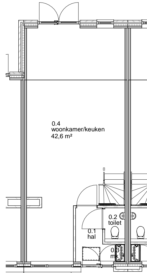
Begane grond
