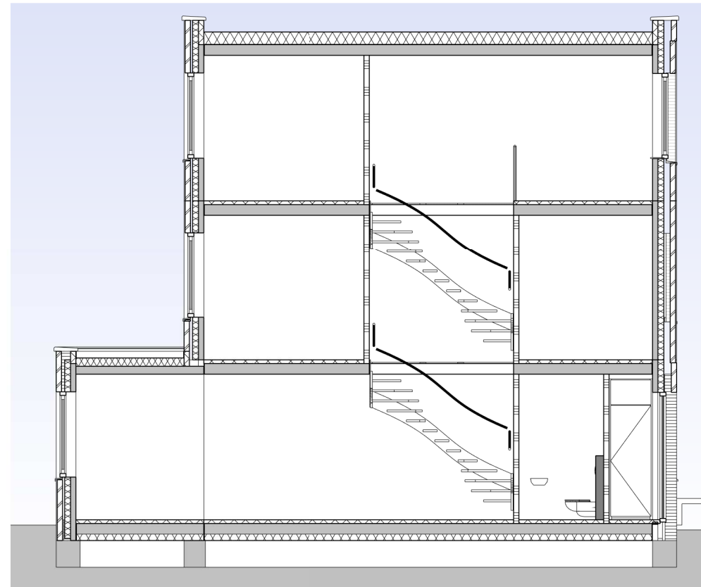
Doorsnede A-A
